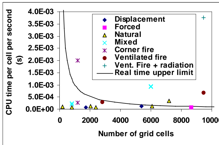
Figure 45. CPU time per cell per second.
